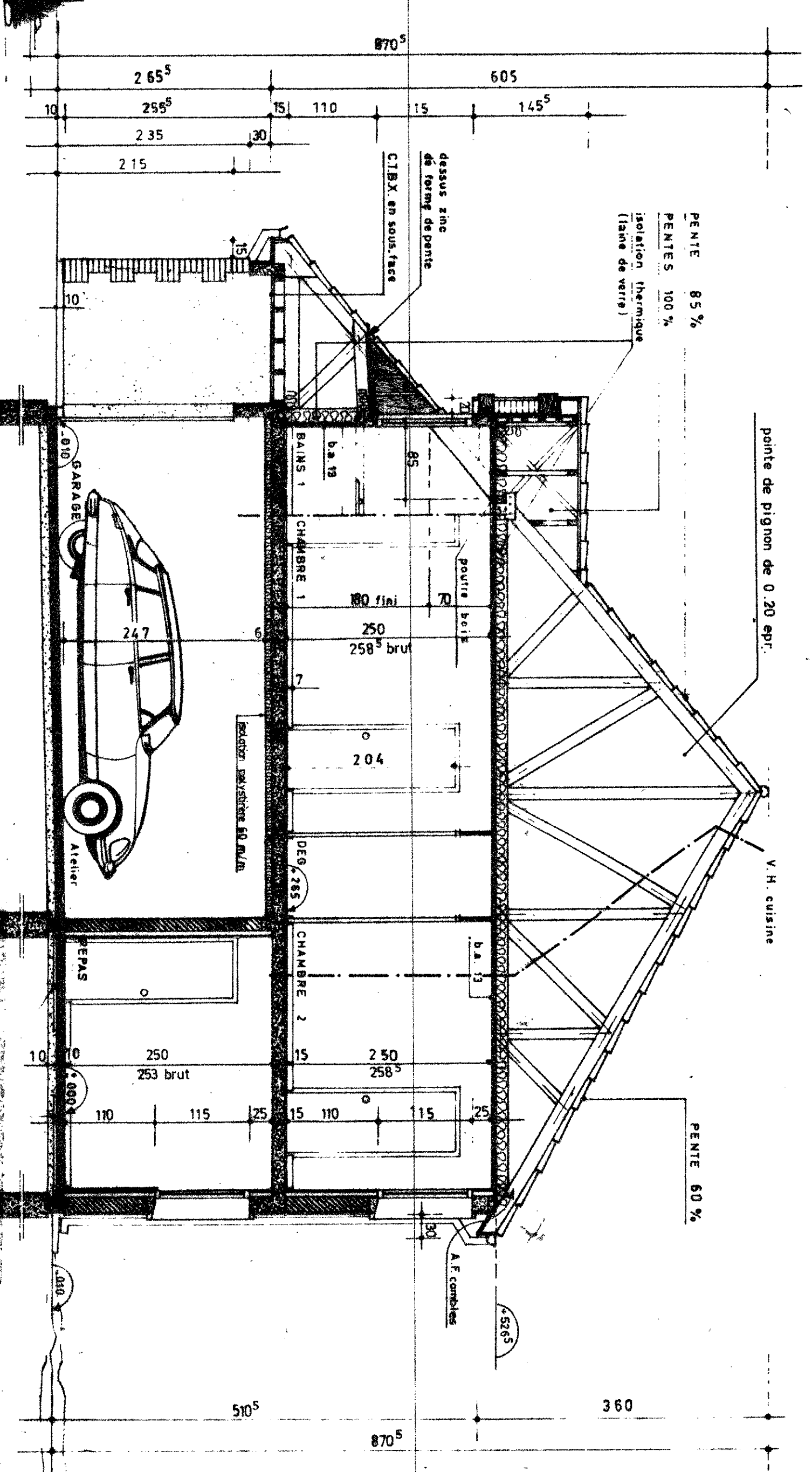
COUPE AA
